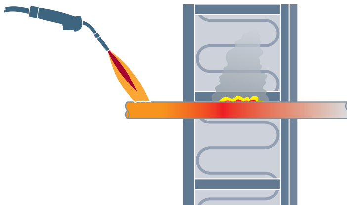
■ Figur 3 Ledning via metallrør til brennbart materiale i en konstruksjon.
