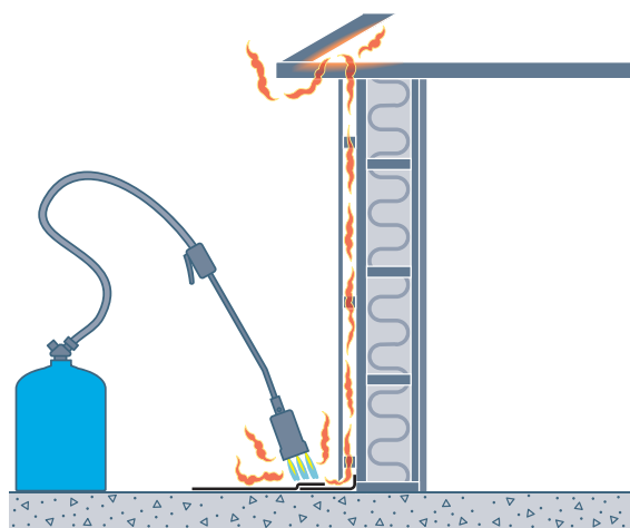
■ Figur 5 Strømning av varme gasser inn i hulrom med brennbart material
